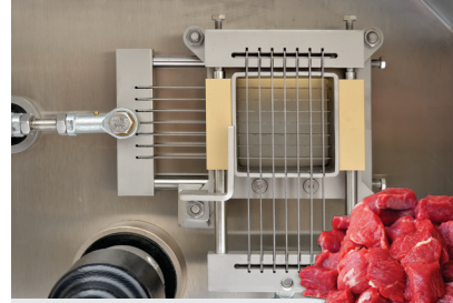
Sebze Doğrama İşkembe Bıçakarası Kuşbaşı Doğrama Tantuni - Ciğer - Çöp Şiş
