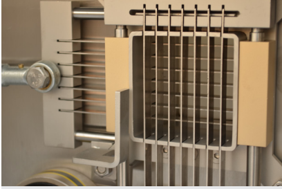
Kolay deęişebilir bıçak sistemi Easy replaceble blade system
